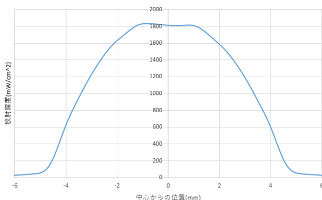
LEDヘッド \phi 10mm時の放射パワー
