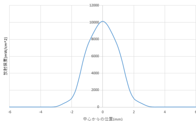
LEDヘッド \phi 3mm時の放射パワー
